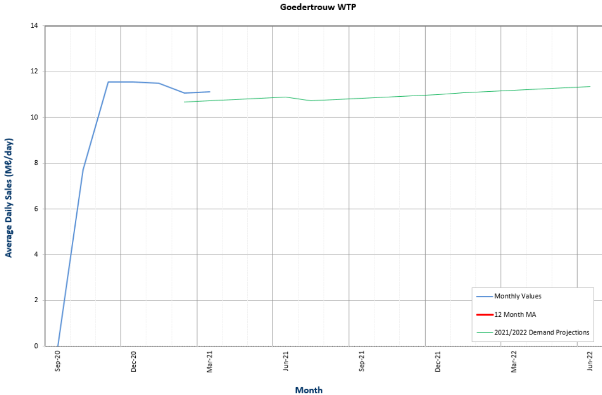
Figure 16.29 Water demand for Goedertrouw WTP
